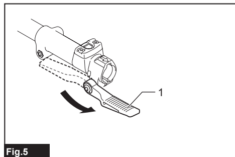
Fig. 5 ► 1. Palanca
